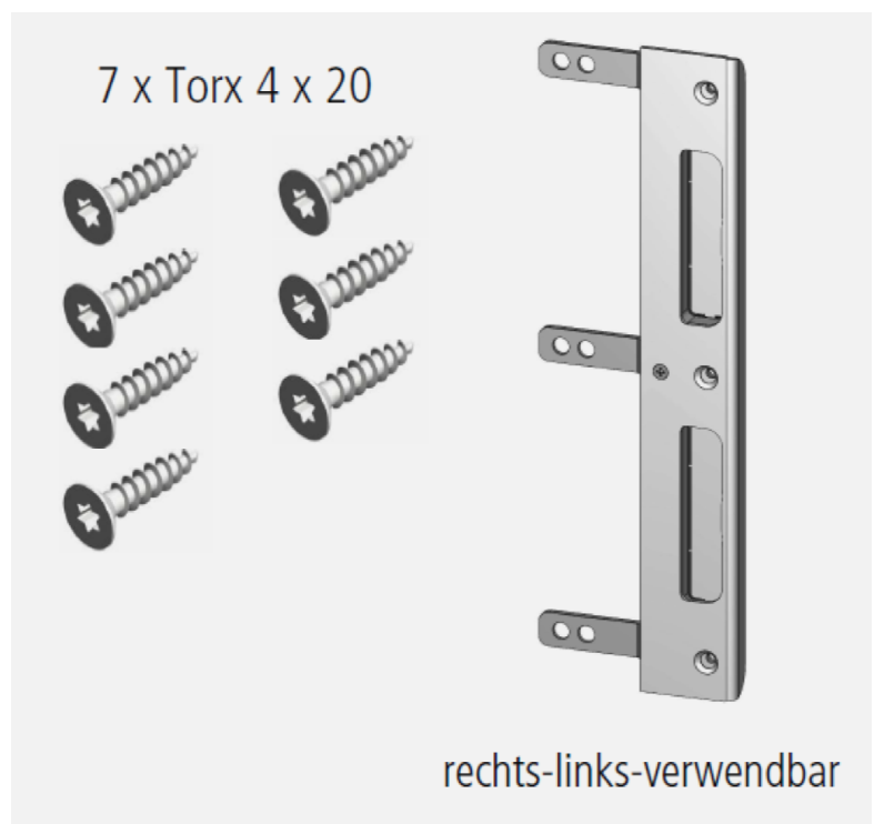
Grauhoff Austauschset WE- Schließblech für Standard- Zargen
