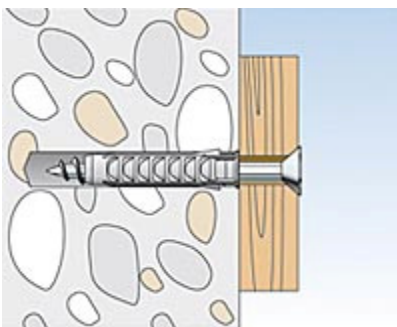
Kunststoff- Spreizdübel SX mit Rand
