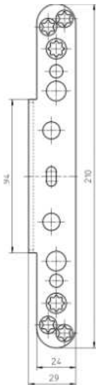
SIMONSWERK VARIANT VX2560KK
