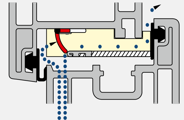
Regel-air® FFL Klappe geschlossen
