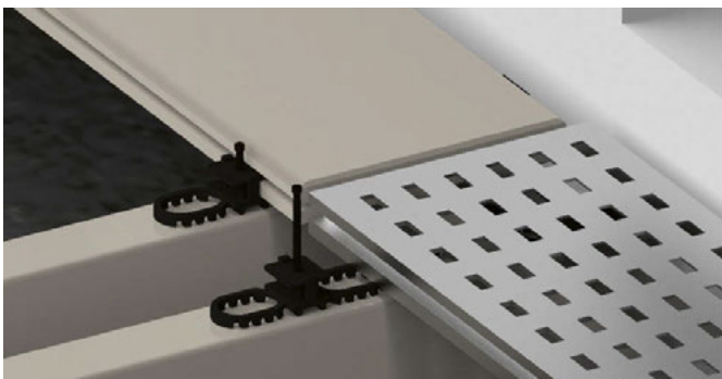
Bild 25. Das Drainageprofil kann auf den Start-Clip geschoben werden und sollte ca. 8 mm Abstand zu den Enden der Dielen haben. Anschließend wird der RASK-Clip unter das Profil geschoben und der Start-Clip kann arretiert werden und das Profil ist damit fixiert.
