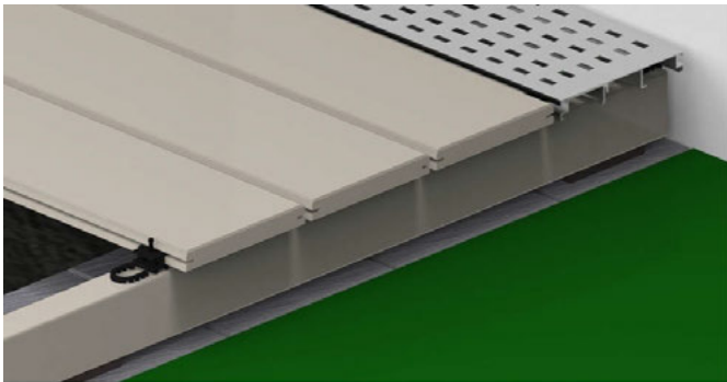
Bild 29. Alle Dielen müssen immer rechtwinklig an beiden Enden abgeschnitten und gerundet oder gefast werden. Bei Bedarf sollten die Brettenden mit SAICOS Stirnkanten-Wachs 8131K behandelt werden. Die Dielen sollten max. 20 mm über die äußere Unterkonstruktion überstehen.
