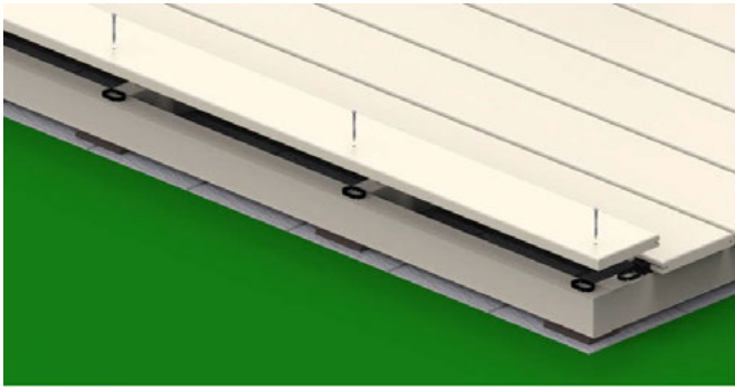
Bild 33. Schneiden Sie bei der letzten Terrassendiele immer auf einer Seite die Nut ab. Wenn die Diele nicht auf die erforderliche Breite geschnitten wird, kann die obere Nutwanne während der Nutzung leicht abbrechen.
