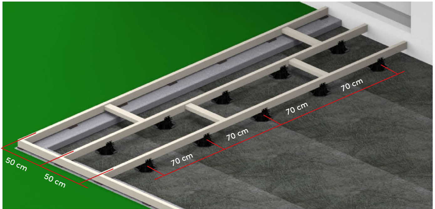
Bild 6. Die Verstellfüße müssen nach den Vorgaben der Hersteller an den Unterkonstruktionen angeschraubt werden. Falls von den Herstellern keine anderslautenden Angaben gemacht werden, sollten maximal 70 cm Achsabstand in Längsrichtung der Balken nicht überschritten werden.
