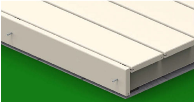
Bild 39. Die Blende sollte mit der Oberkante der Terrassendielen abschließen und die Befestigung muss mit min. V2A Terrassenschrauben erfolgen.
