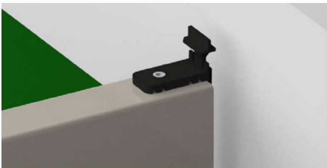
Bild 19. Nachdem das Unterteil vom Start-Clip verschraubt ist, stecken Sie bitte das Oberteil mit der Feder nach vorne bis zur ersten Arretierung in das Unterteil.
