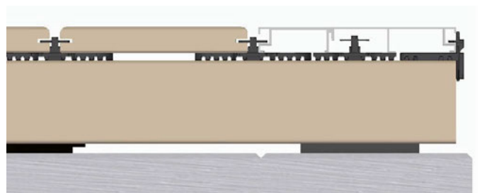
Bild 26. Die eingekürzten RASK-Clips stellen sicher, dass das Drainageprofil an allen Stellen stabil unterstützt wird und sich bei Belastung nicht durchbiegen kann. Die Fixierung des Drainageprofil erfolgt an der Hausseite mit dem Start-Clip und dem RASK-Clip auf der Dielenseite.
