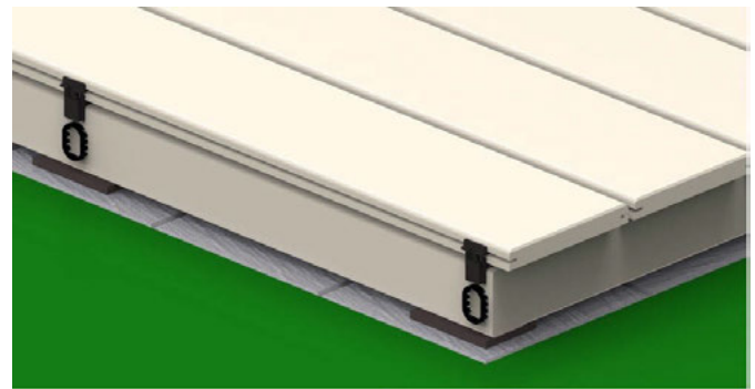
Bild 38. Da die vordere genutete Kante der Terrassendiele sehr bruchempfindlich ist, muss immer eine Blende montiert werden. Für die Montage der Blende verwenden Sie wieder Teilstücke vom RASKCLIP. Diese Teilstücke stellen den richtigen Abstand sicher.
