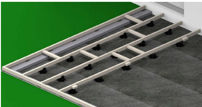
Bild 10. Drei kurze Abschnitte 38 x 68 ca. 100 mm lang, werden zuerst flachliegend an den ersten Balken geschraubt. Die Stücke sollten ca. 10 mm tiefer liegen.
