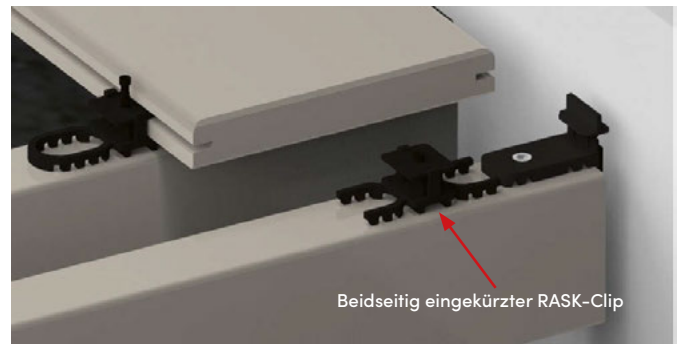
Bild 24. Für die Drainagerinne müssen zusätzlich auf jeder Unterkonstruktion ein beidseitig eingekürzter RASK-Clip montiert werden. Mit einem z. B. Seitenschneider ist das einfach machbar. Der RASK-Clip kann komplett festgeschraubt werden.
