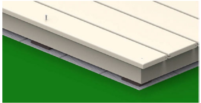
Bild 34. Schieben Sie die abgeschnittene Terrassendiele mit der Nutseite auf die RASK-Clipse. Anschließend wird die Diele mit einer Terrassenschraube min. 5 x 60 V2A alle 50 cm auf der Unterkonstruktion verschraubt. Die Schrauben sollten gleichmäßig max. 1 mm tief versenkt werden.
