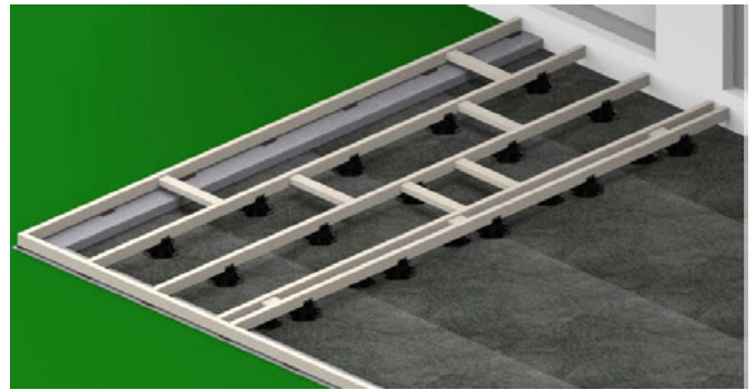
Bild 11. Danach wird der 2 Balken inkl. der Verstellfüße an die 3 kurzen Balken angeschraubt.
