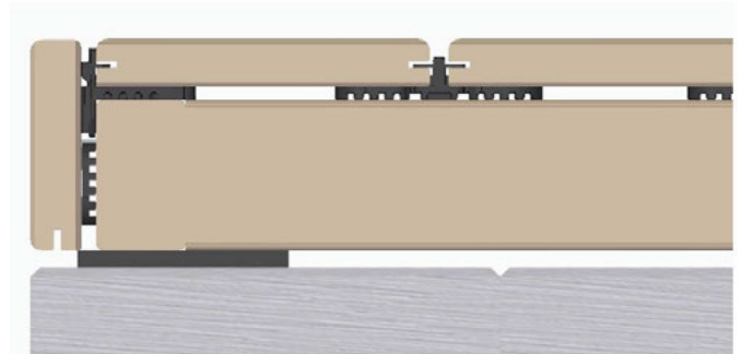
Bild 40. Unterhalb der Blende sollte min. 8 mm Luft eingeplant werden.
