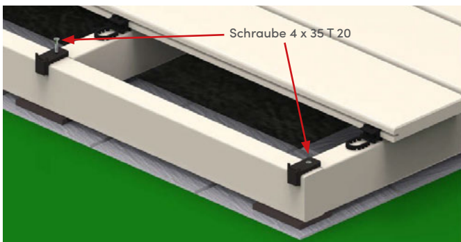
Bild 35. Zuerst wird nur das Unterteil vom Startclip mit den Schrauben 4 x 35 mm (T 20) auf die vordere Holzunterkonstruktion geschraubt.
