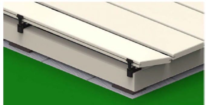
Bild 36. Die Diele wird danach schräg auf den RASK-Clip geschoben und anschließend können die Oberteile in die Nut der Diele gesteckt werden.
