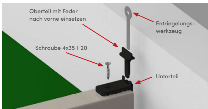
Bild 17. Der Start-Clip besteht aus einem Unterteil und einem Oberteil und wird nicht zusammengebaut geliefert. Sie können zuerst nur die Unterteile auf die Unterkonstruktionen verschrauben.
