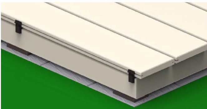
Bild 37. Wenn alle Oberteile eingesteckt sind, muss die Terrassendiele runtergedrückt werden und dadurch wird das Oberenteil vom Startclip arretiert.
