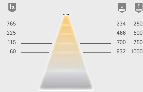
Lichtverteilungsdiagramm 50°
