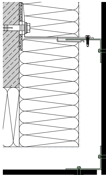
Außenecke A105
