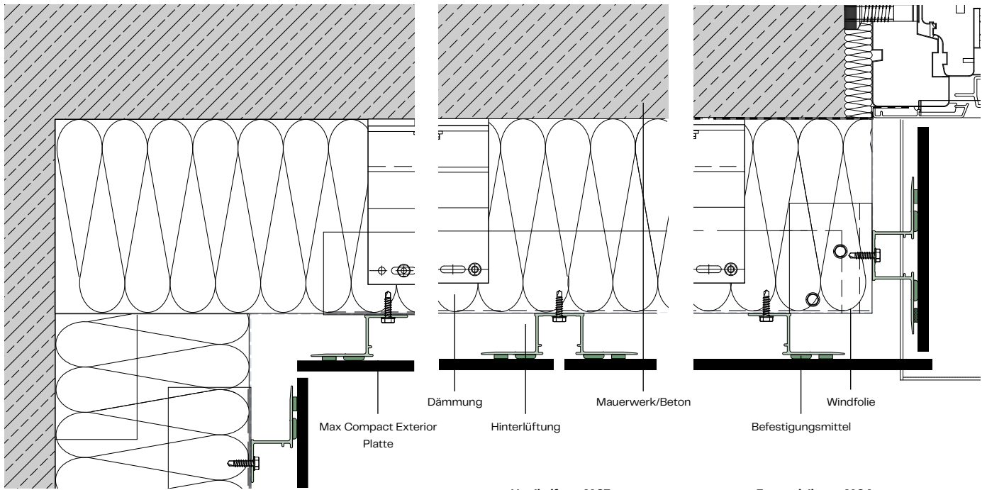
Innenecke A106
