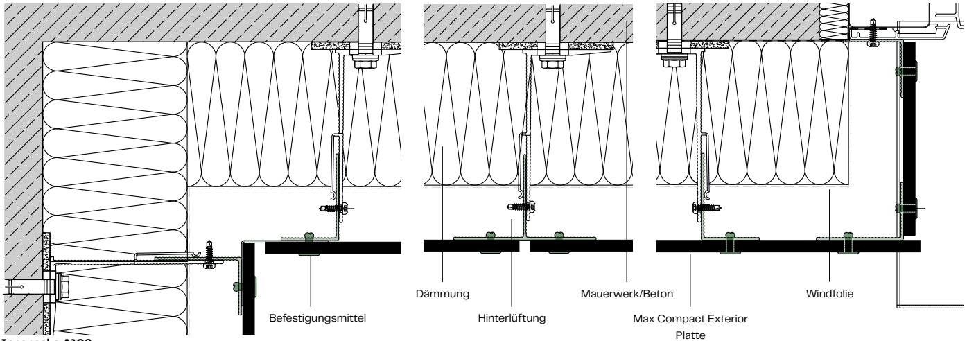
Innenecke A106
