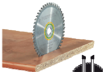
Feinzahn- Sägeblatt 160x2,2x20 W48
