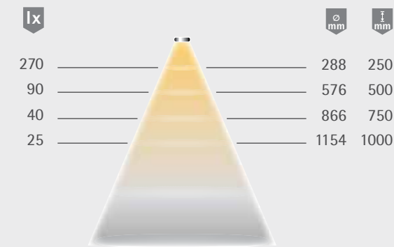
Lichtverteilungsdiagramm 60°
