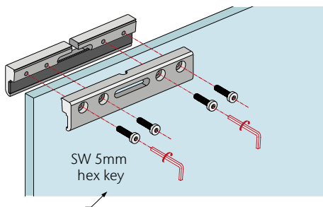
Glastür A / Glass door A / Porte vitrée A
