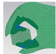
Zangenschlüssel: spielfreie Flächenpressung
