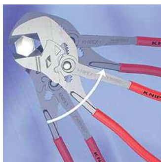
Arbeiten nach dem Ratschenprinzip
