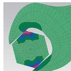
Herkömmlicher Schraubenschlüssel: Kantenpressung führt zu Beschädigung
