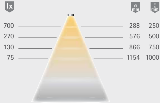
Lichtverteilungsdiagramm 60°
