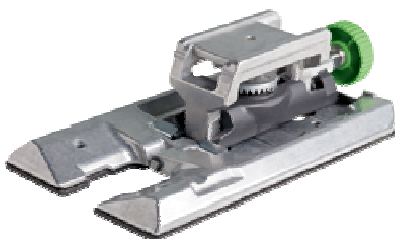
Winkeltisch WT- PS400
