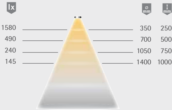
Lichtverteilungsdiagramm 60°
